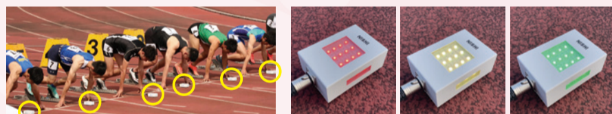
スタート合図を光で伝える装置 赤「On your marks」⇒黄「Set」⇒緑「Bang!」
